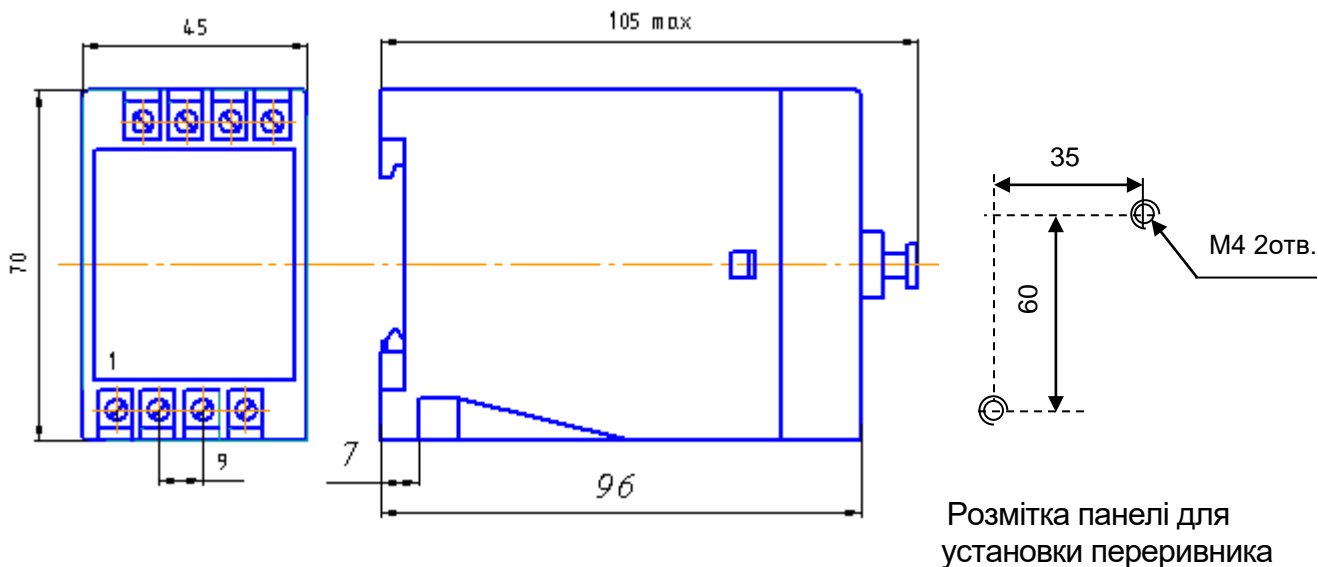
Рисунок 2 – Загальний вигляд переривника
