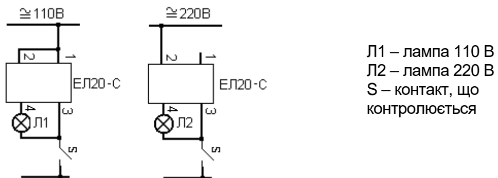
Рисунок 1 – Схема застосування переривника
