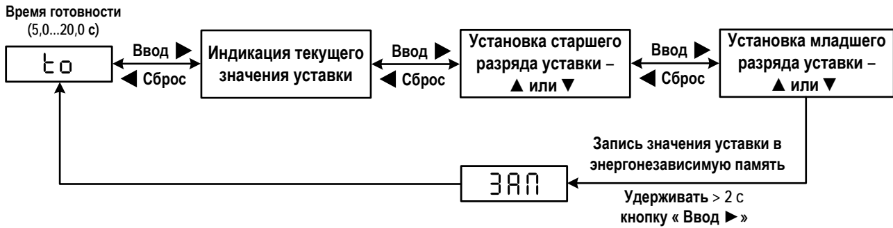
Рисунок 8 – Программирование времени готовности
