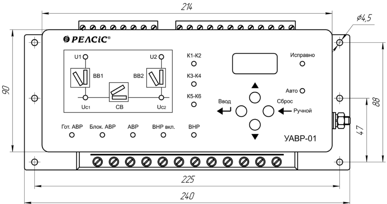
Рисунок 2 - Внешний вид и габаритные размеры устройства УАВР-01
