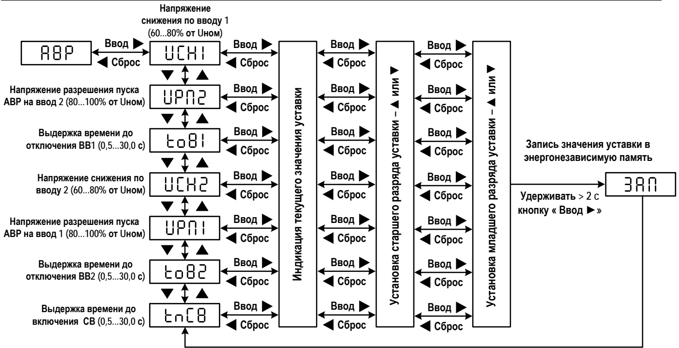
Рисунок 6 – Программирование уставок АВР
