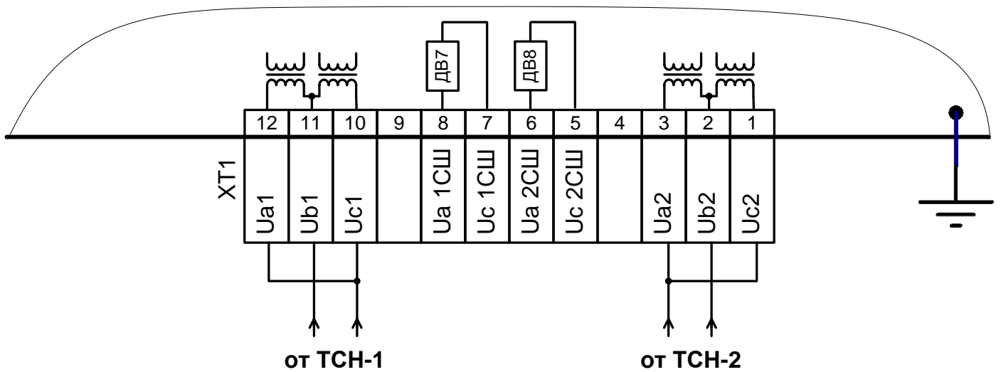
Рисунок 4 – Схема подключения устройства УАВР-01 при использовании на объекте с однофазными трансформаторами ТСН-1(2)
