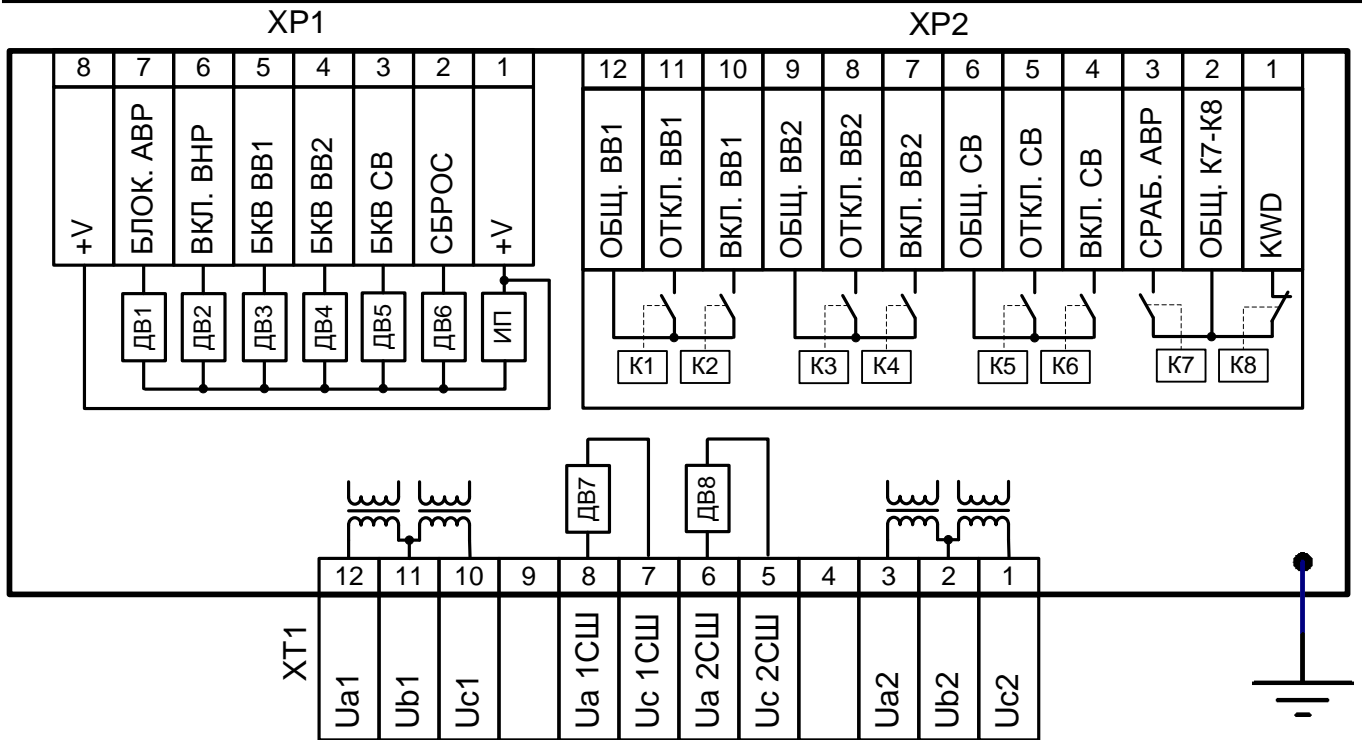
Рисунок 3 - Маркировка разъемов устройства УАВР-01
