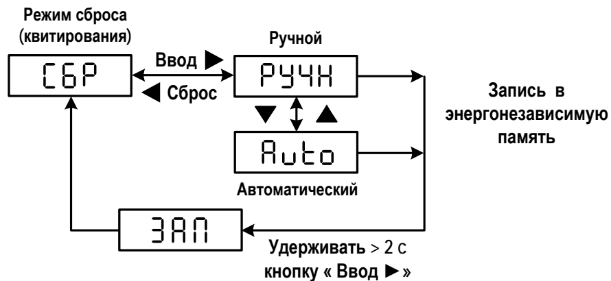
Рисунок 9 – Программирование режима сброса
