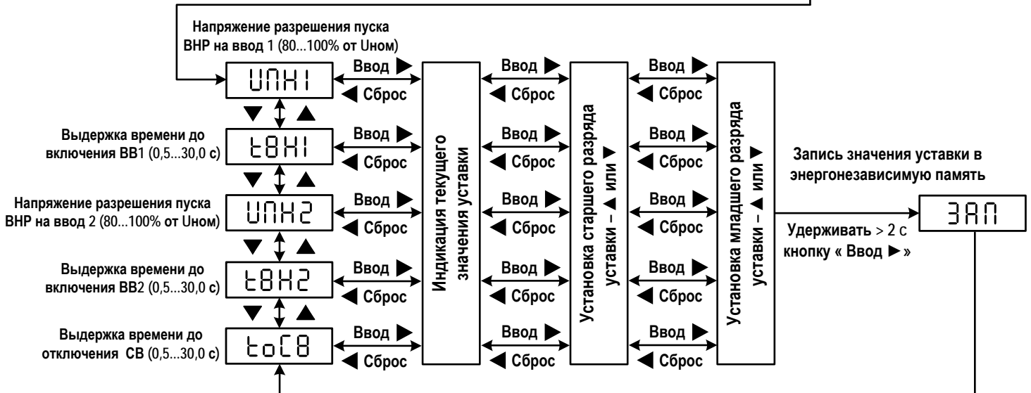
Рисунок 7 – Программирование уставок ВНР
