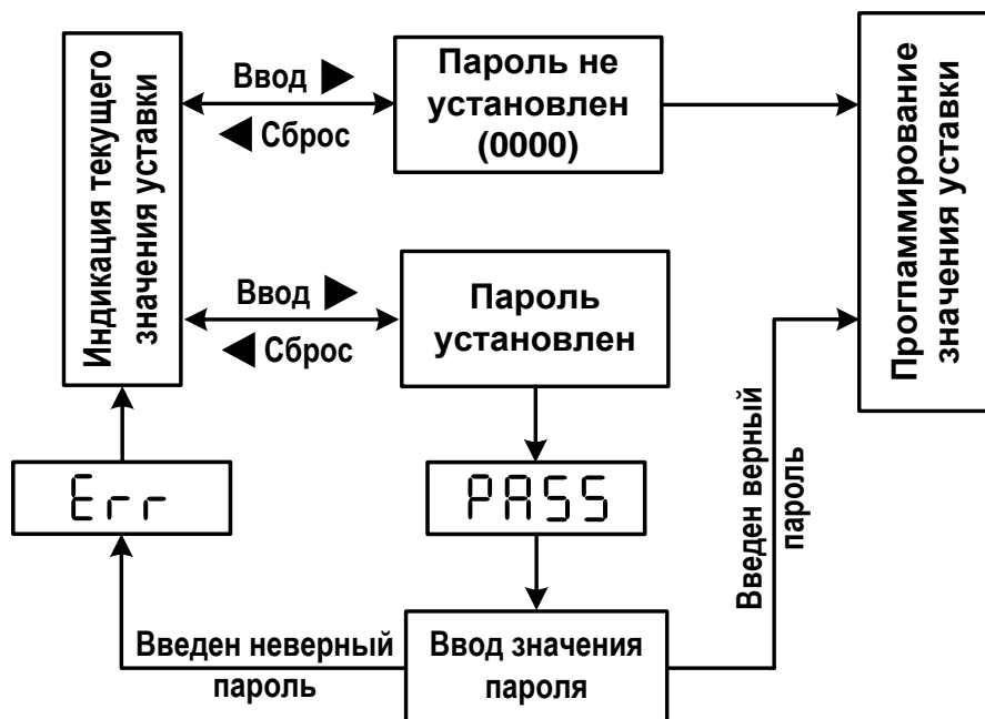
Рисунок 10 – Алгоритм действия пароля
