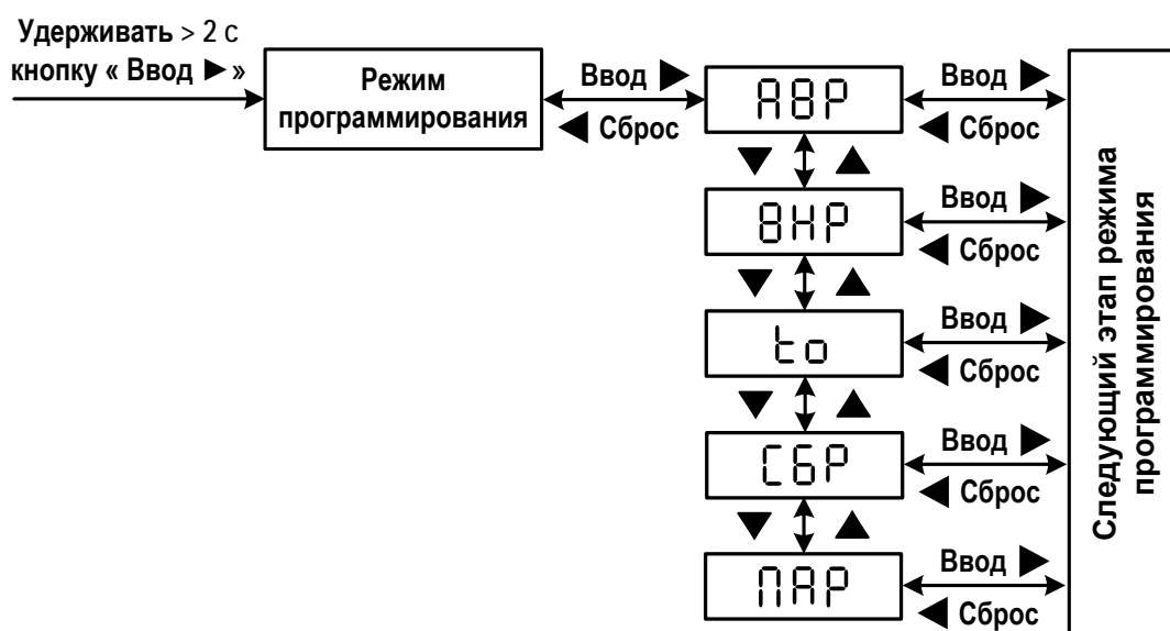
Рисунок 5 – Вход в режим программирования
