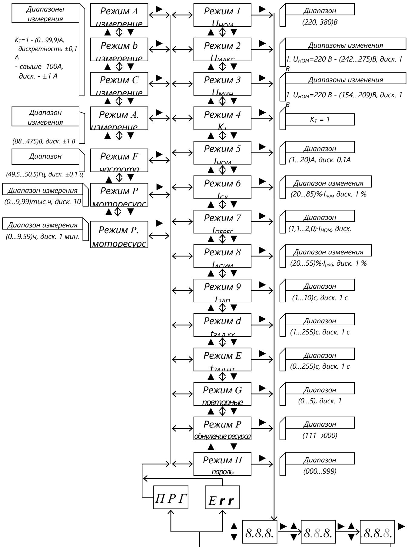
Рисунок 6 - Алгоритм функционирования реле защиты двигателя РДЦ-01-203
