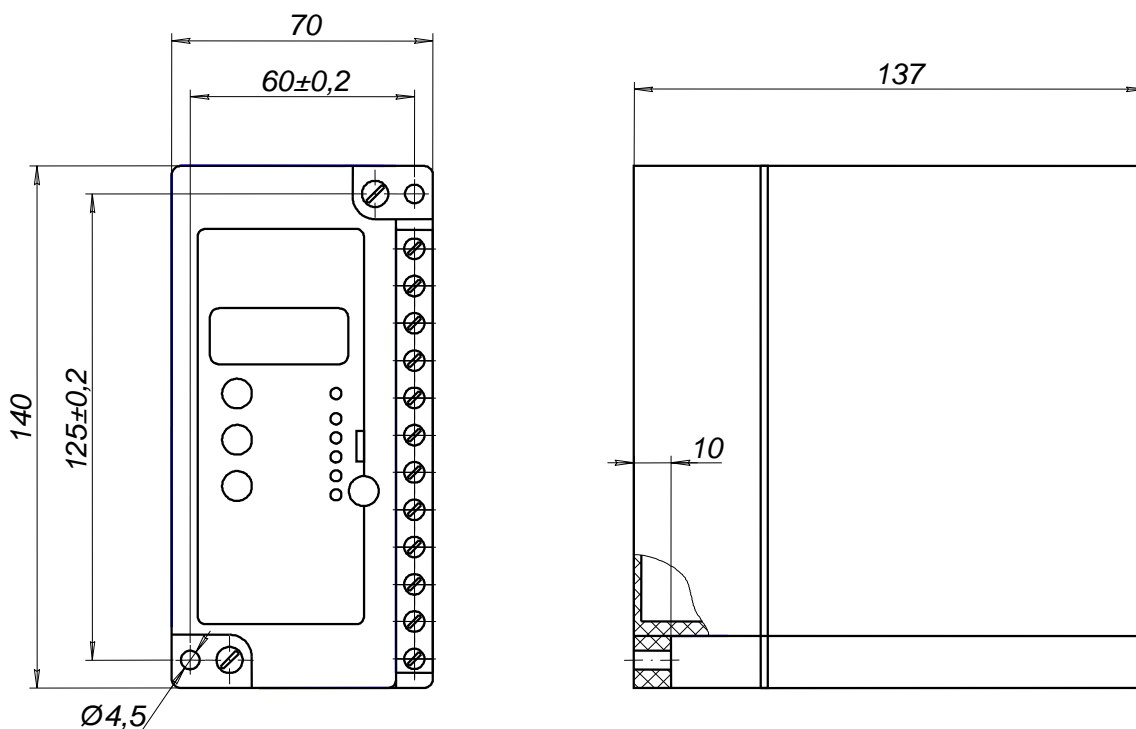
Рисунок 1 - Габаритные и установочные размеры реле РДЦ-01-203
