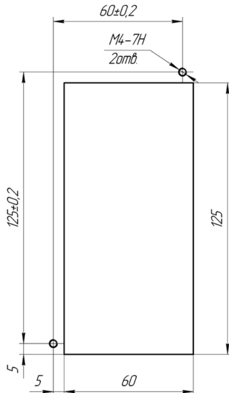
Рисунок 6 – Разметка панели для заднего присоединения проводов РДЦ-01-057-4,5
